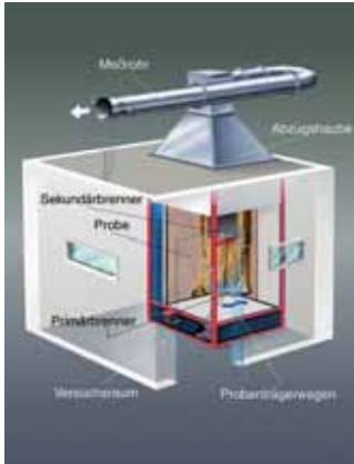
DIN EN 20187 normuna göre deneysel kurulum
